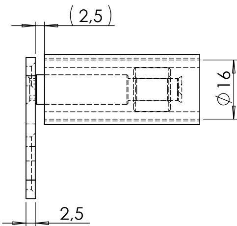
DETAIL A MAßSTAB 1 : 1
